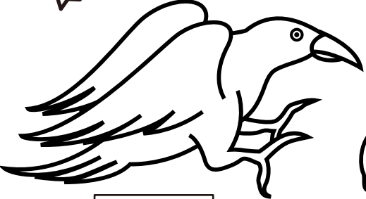
からす座
