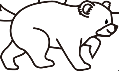
こぐま座
